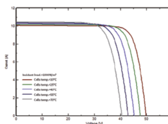
不同工作温度下I-V曲线 (SPP415DH7H)
