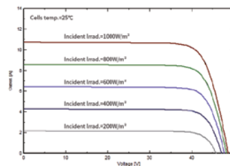
不同辐照度下I-V曲线 (SPP415DH7H)
