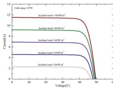
不同辐照度下 I-V 曲线 (SSP450QH7H)
