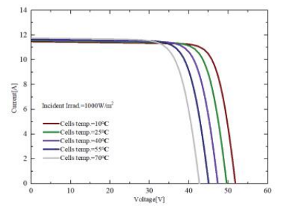
不同工作温度下 I-V 曲线 (SSP450QH7H)
