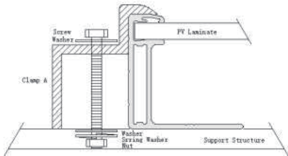
Clamp A at the module edge
