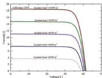
不同辐照度下 I-V 曲线 (SSD600YH6H)
