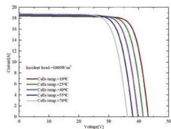
不同工作温度下 I-V 曲线 (SSD600YH6H)
