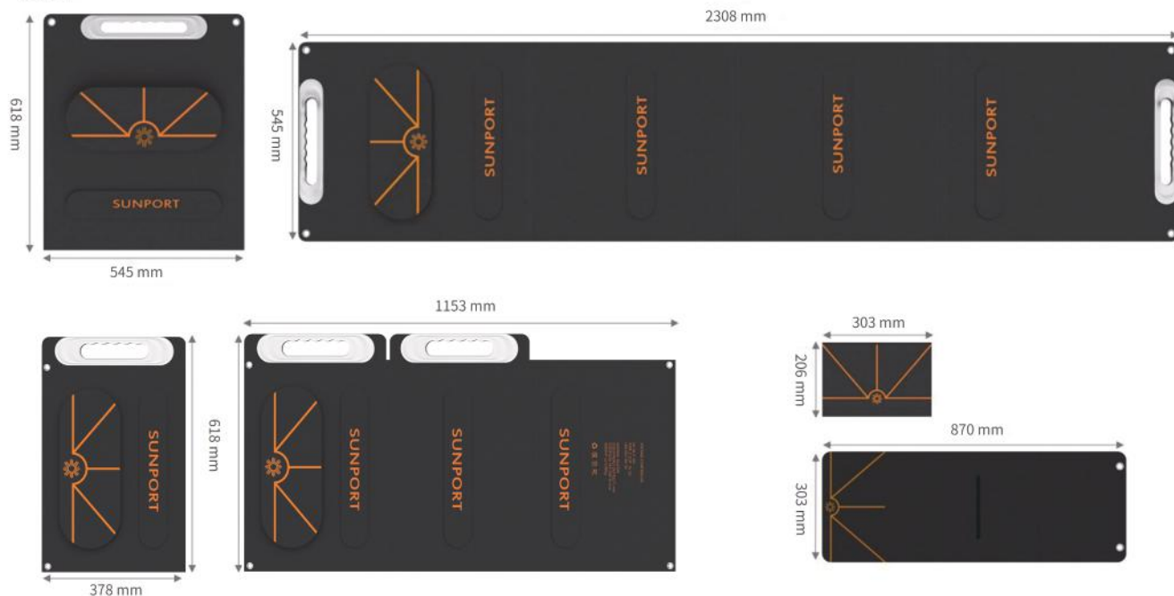
尺寸图
